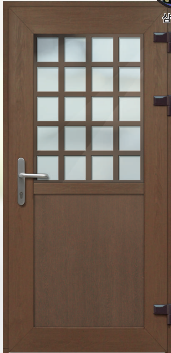
DOD 5241 사이즈 W1000×H2100 W900×H2100 돌출형 도어 클로저 사용
